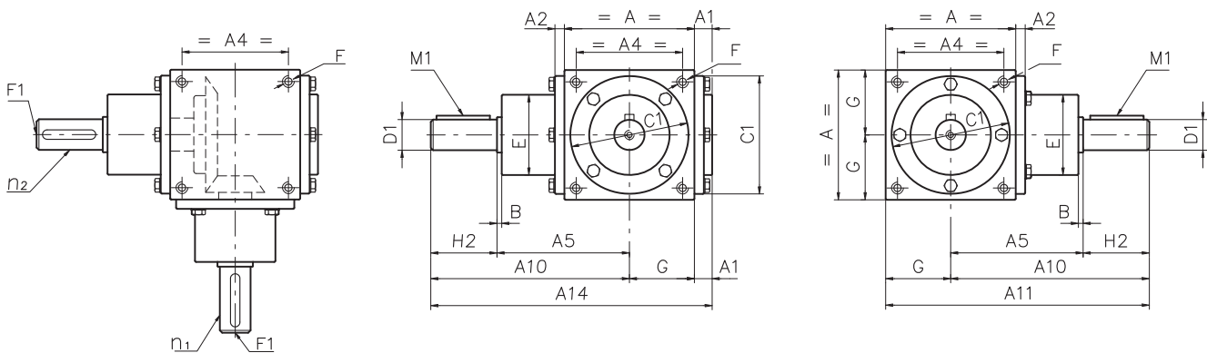
Rozměry [mm]
